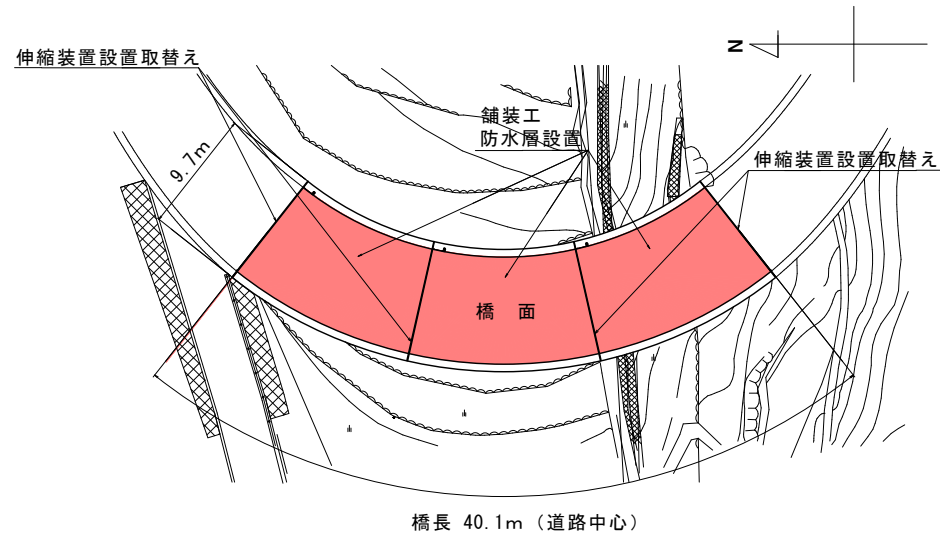
平面図
