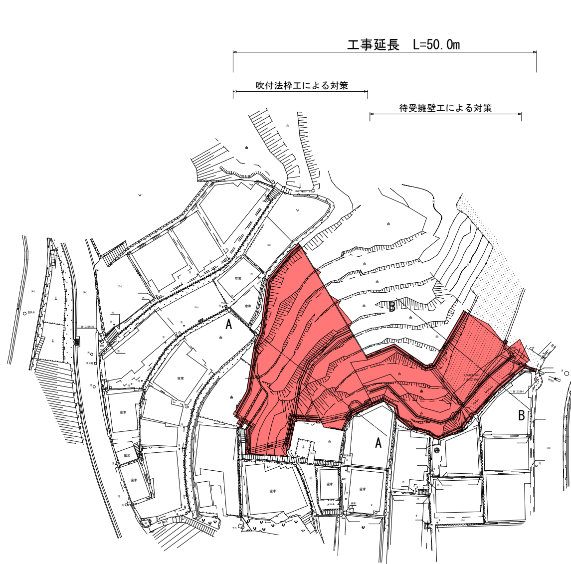
平面図
